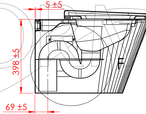
KESIT A-A
