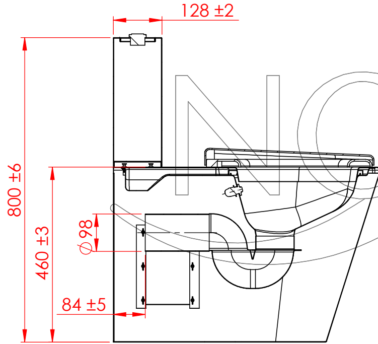
KESIT J-J ÖLÇEK 1 : 10
