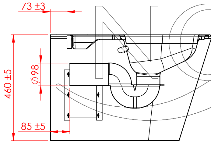
KESIT B-B ÖLÇEK 1 : 10
