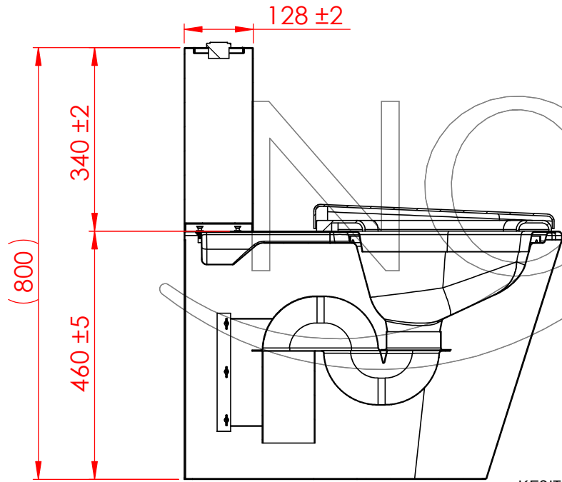
KESIT J-J ÖLÇEK 1 : 10
