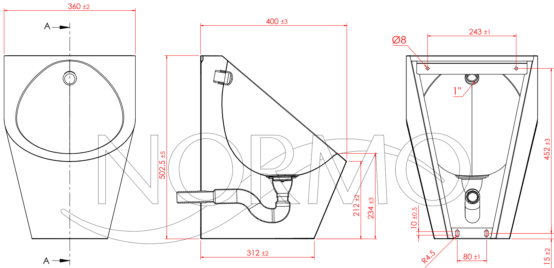
KESIT A-A
